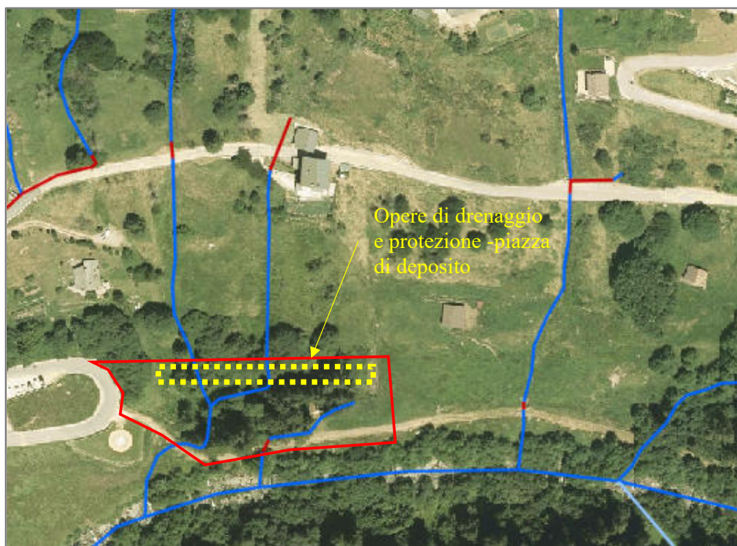
Figura 6.1: Planimetria con individuazione delle opere di mitigazione idrogeologiche.
