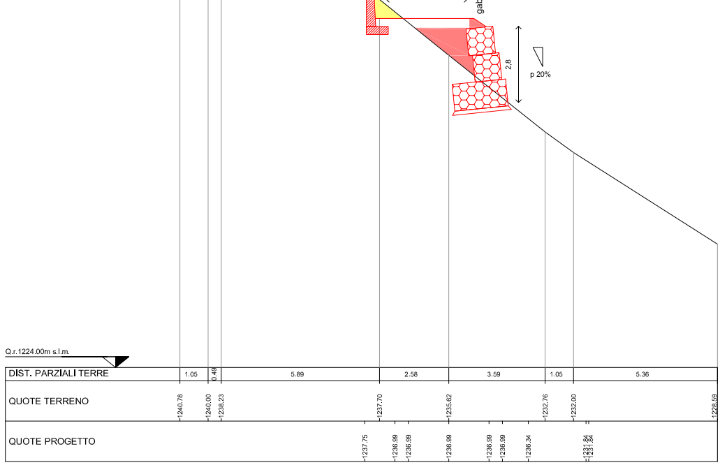
SEZIONE N. 7 DIST.PROG.: 100,00
