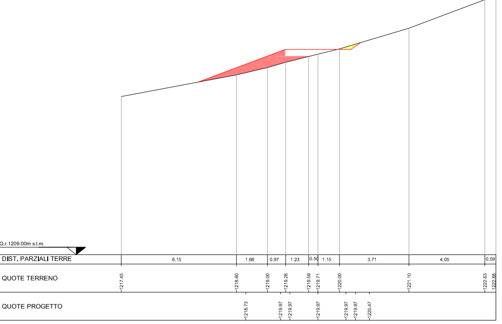
SEZIONE N. 18 DIST.PROG.: 300,00
