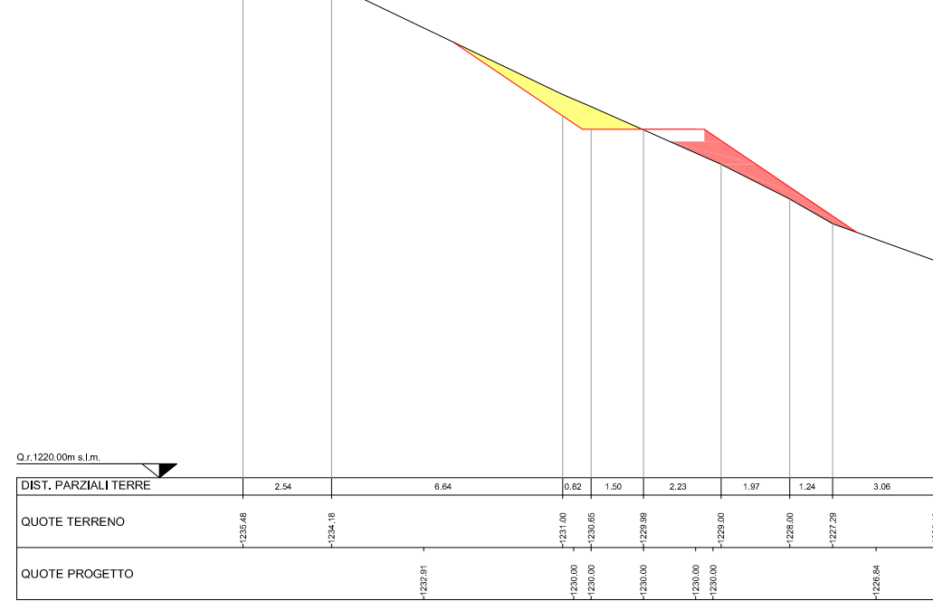
SEZIONE N. 11 DIST.PROG.: 167,00
