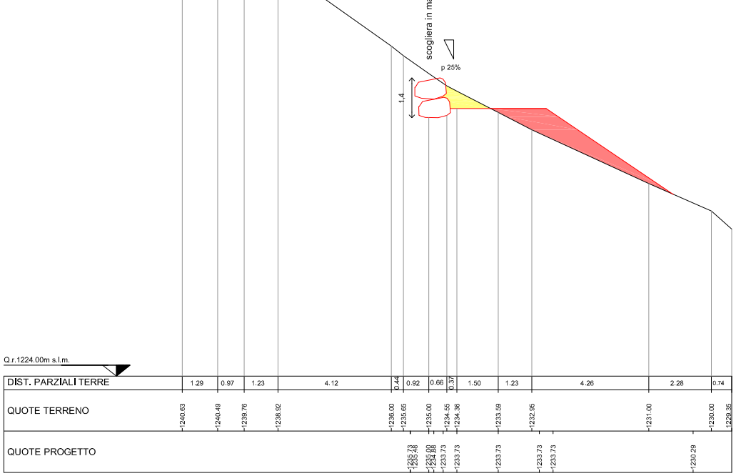
SEZIONE N. 9 DIST.PROG.: 133,00
