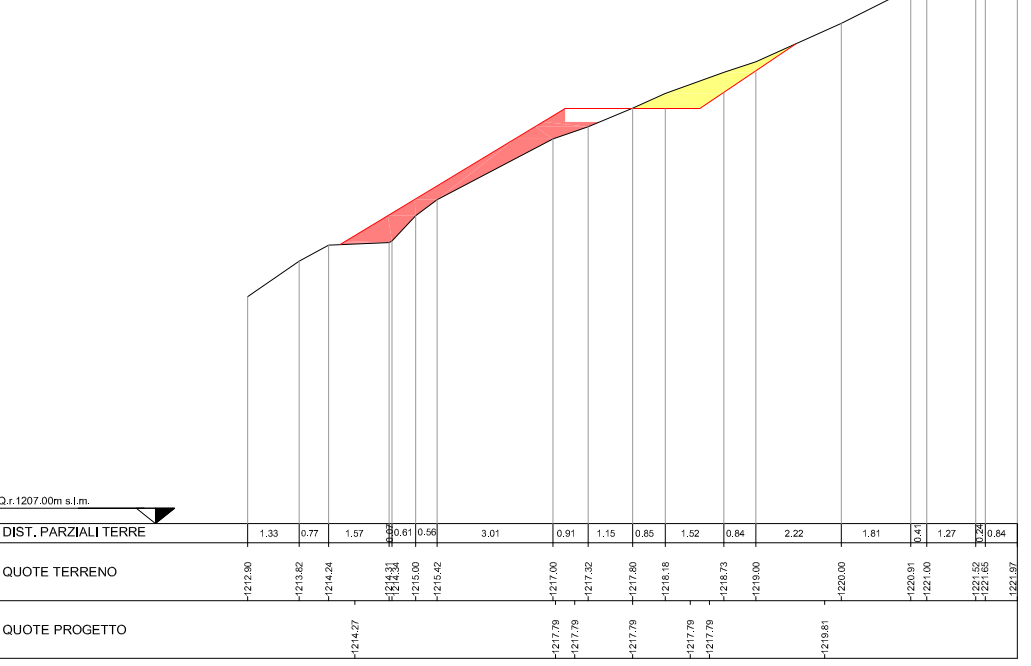
SEZIONE N. 19 DIST.PROG.: 320,00
