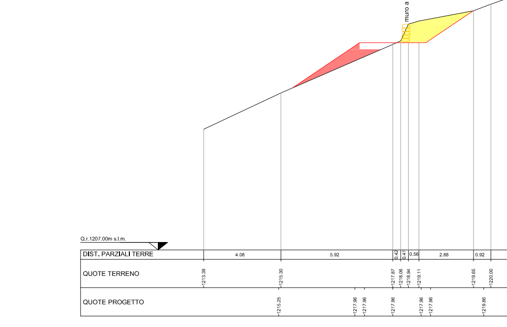
SEZIONE N. 20 DIST.PROG.: 340,00
