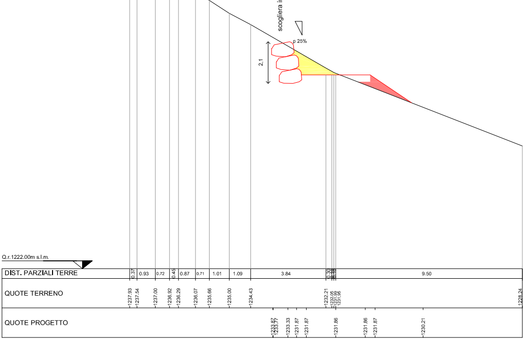
SEZIONE N. 10 DIST.PROG.: 146,00
