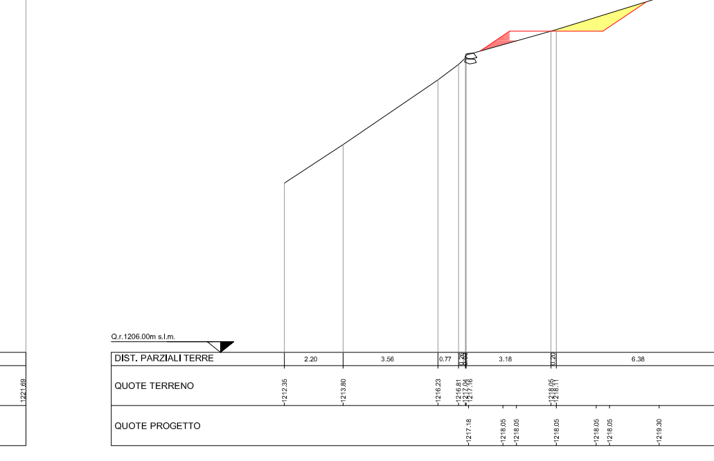
SEZIONE N. 21 DIST.PROG.: 360,00
