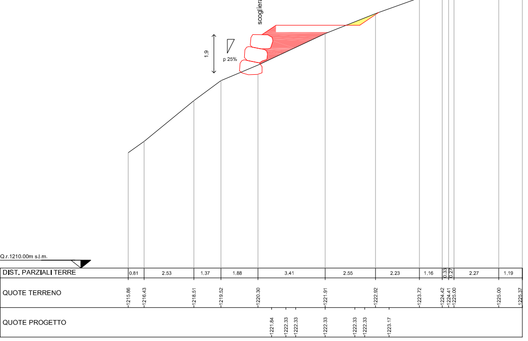
SEZIONE N. 17 DIST.PROG.: 280,00
