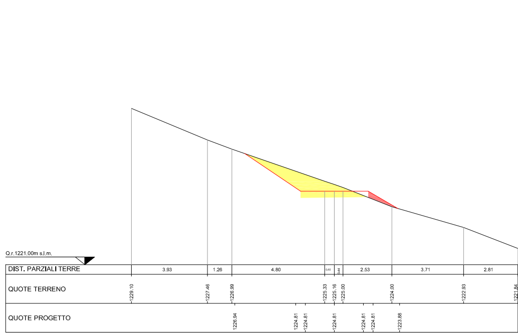
SEZIONE N. 15 DIST.PROG.: 240,00
