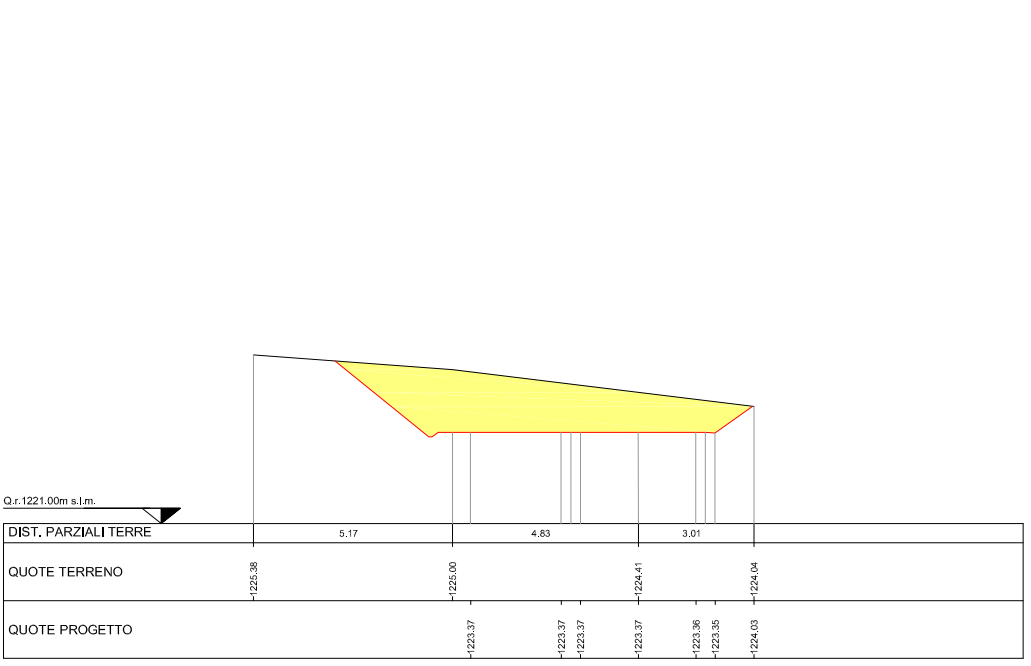
SEZIONE N. 16 DIST.PROG.: 260,00
