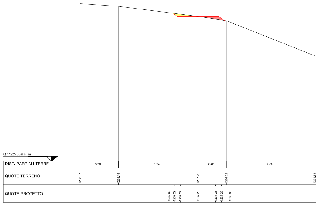
SEZIONE N. 6 DIST.PROG.: 90,00
