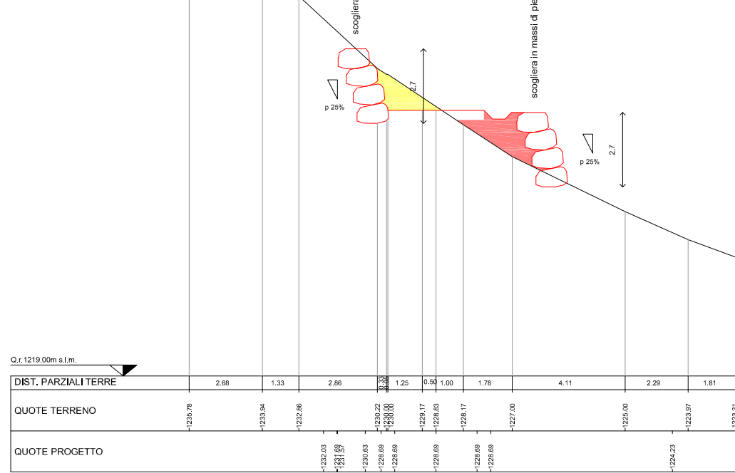
SEZIONE N. 12 DIST.PROG.: 180,00
