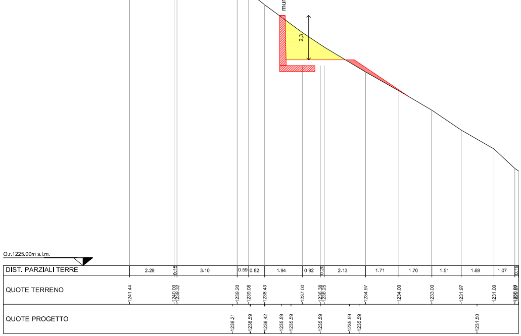
SEZIONE N. 8 DIST.PROG.: 115,00
