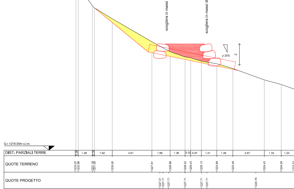
SEZIONE N. 13 DIST.PROG.: 200,00
