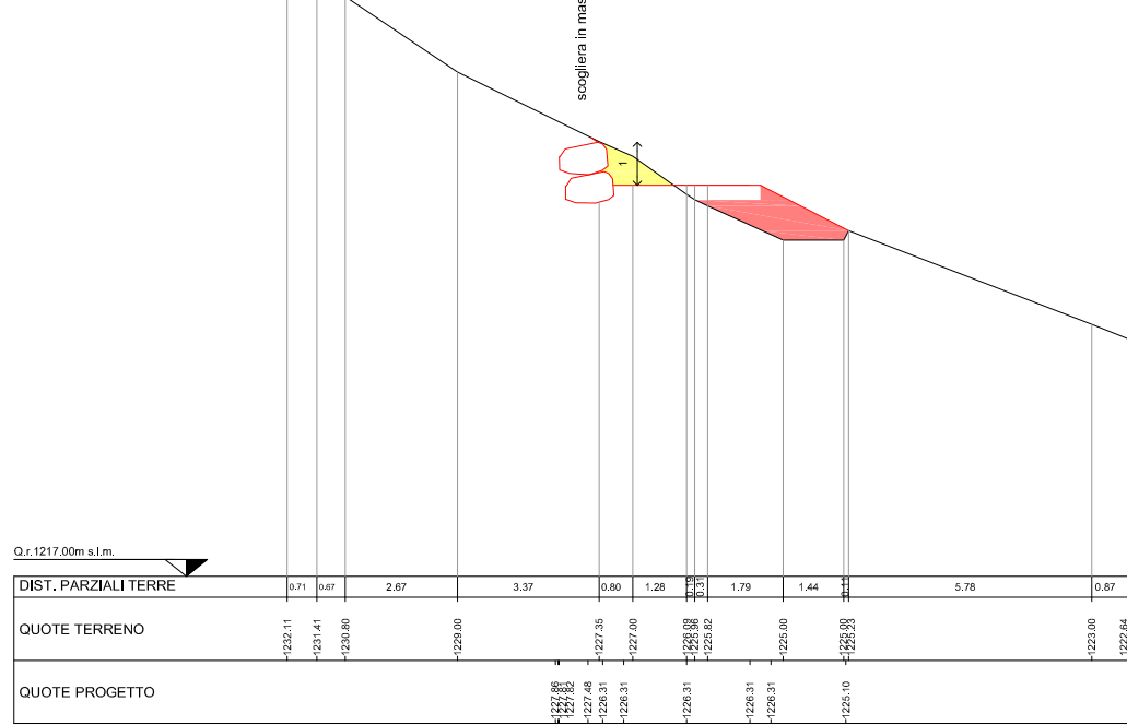
SEZIONE N. 14 DIST.PROG.: 220,00
