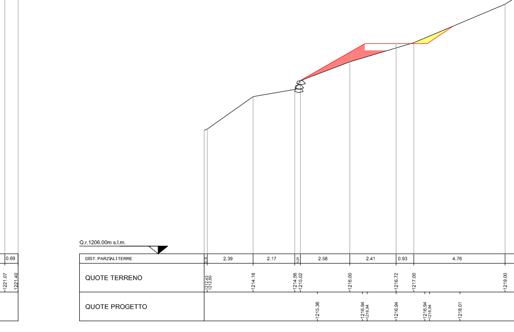
SEZIONE N. 22 DIST.PROG.: 380,00
