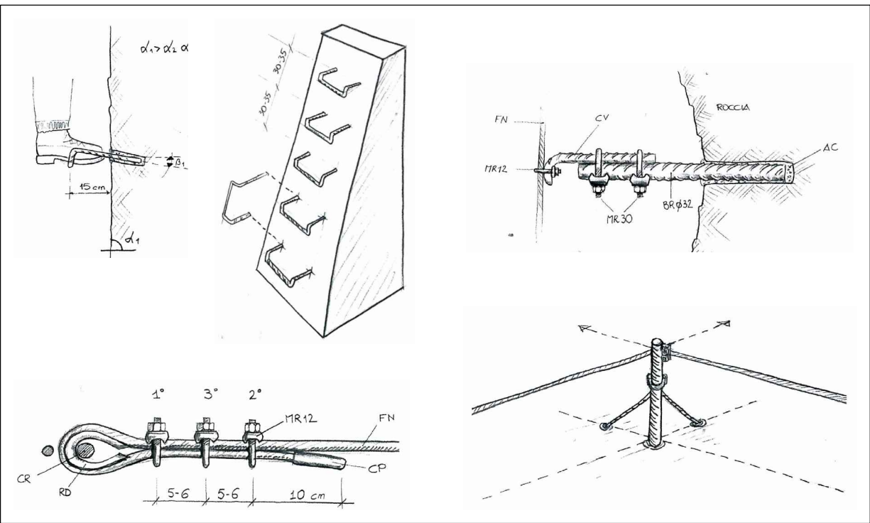
PARTICOLARI - scala a vista
