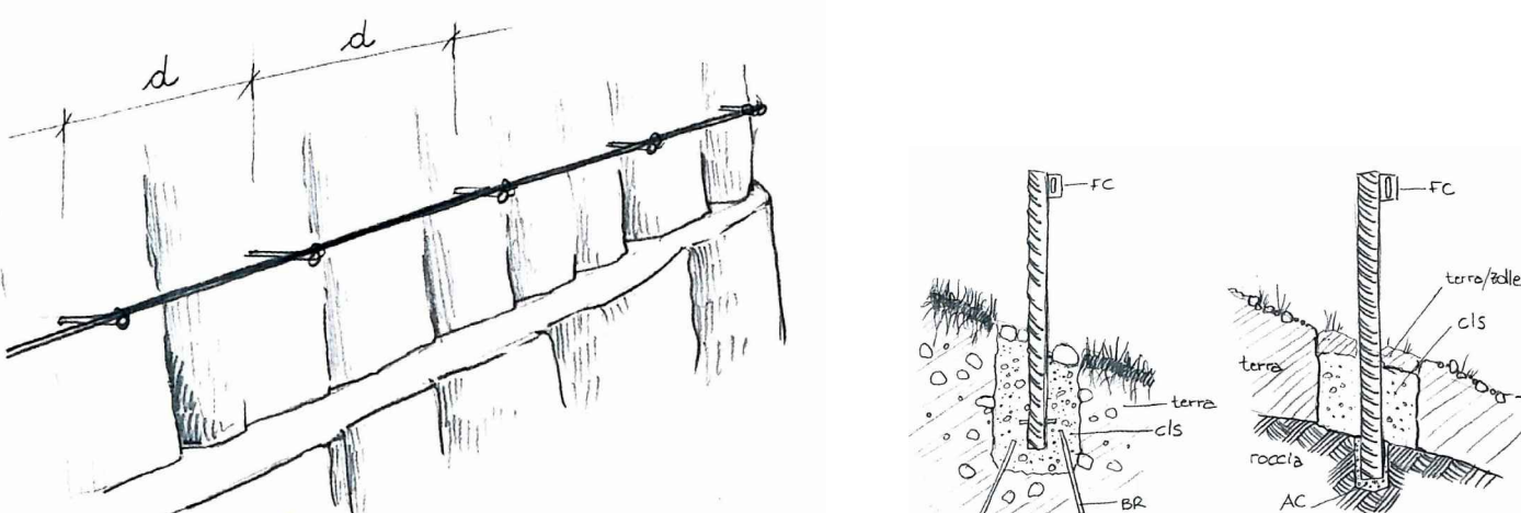
lavorazione TIPO "C" (*)
