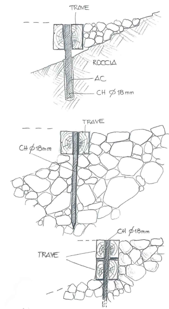
lavorazione TIPO "A" (*)
