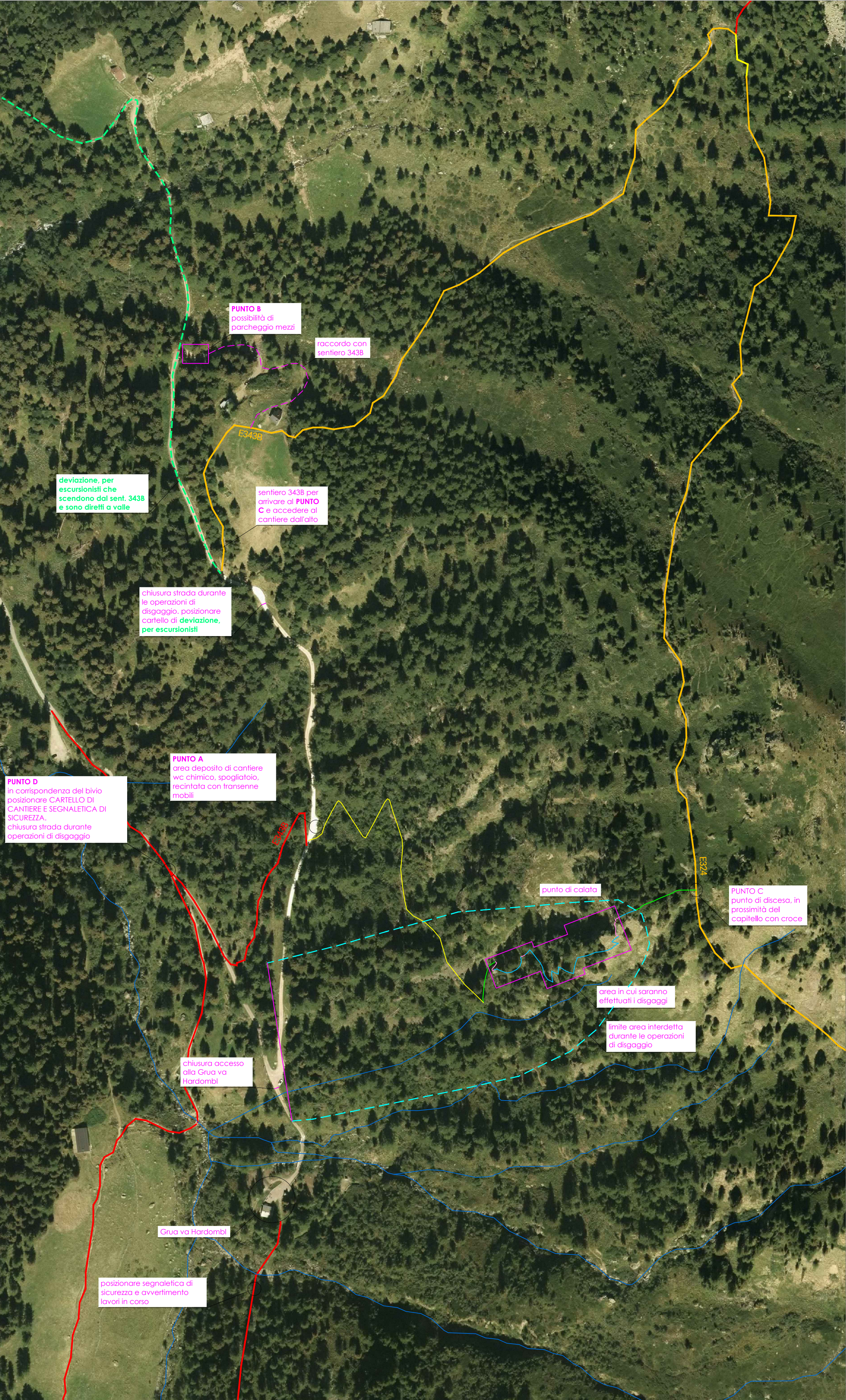
LAYOUT DI CANTIERE - scala 1:2000 (sfondo: Ortofoto PAT 2015)
